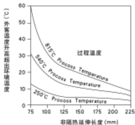
图 1 变送器外壳温度升高与延长件长度的关系
