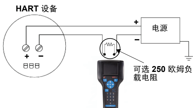
图 3-5. 连接 250 欧姆电阻
