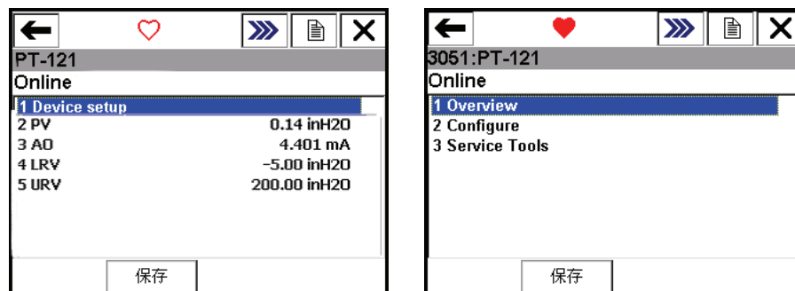
图 3-7. HART 在线菜单和设备仪表盘在线菜单
